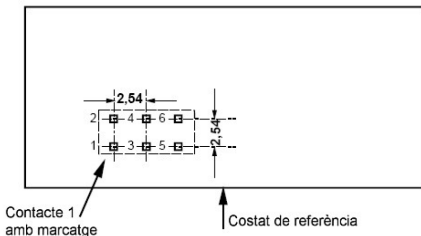
Esquema 1: esquema de posicionament del contacte 1 amb un connector 2 x 3 (versió recta) i numeració dels contactes (1 a filera senar, 2 a filera parell)
